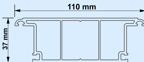
DEROX uPVC DOOR MULLION / DIVIDER
