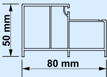
DEROX uPVC DOOR FRAME
