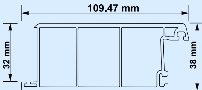
DEROX uPVC DOOR SASH
